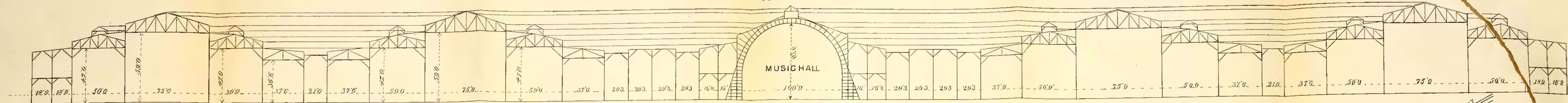
LONGITUDINAL SECTION.
